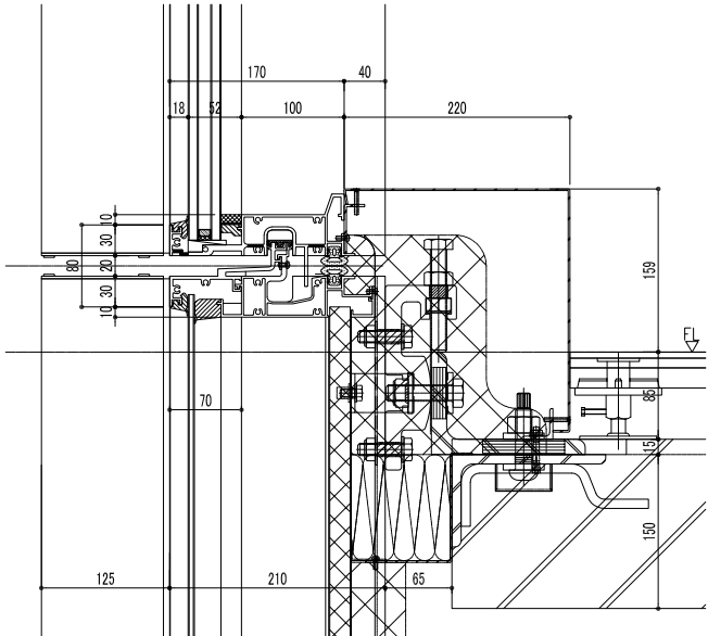
縦断面図 (S=1/8)
