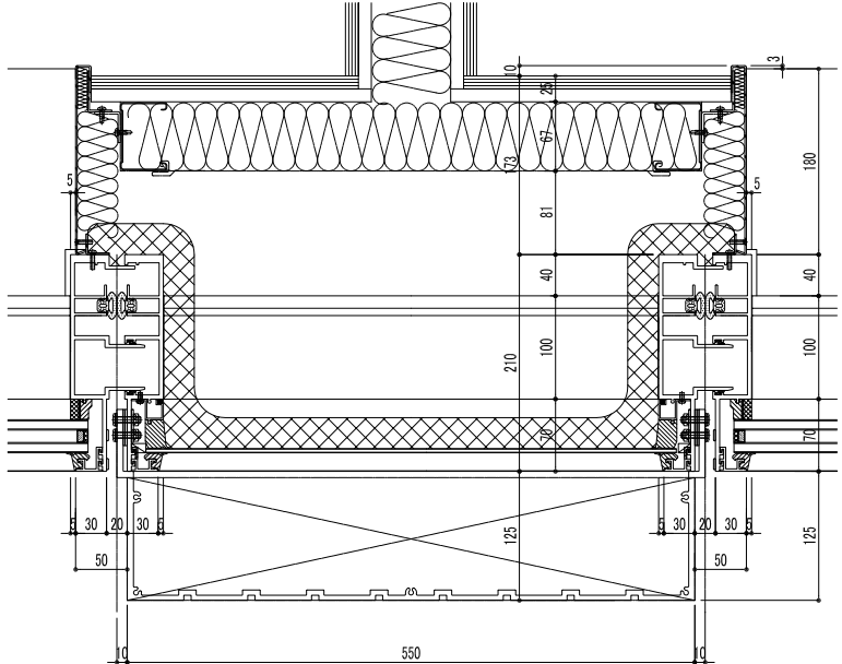
横断面図 (S=1/8)
