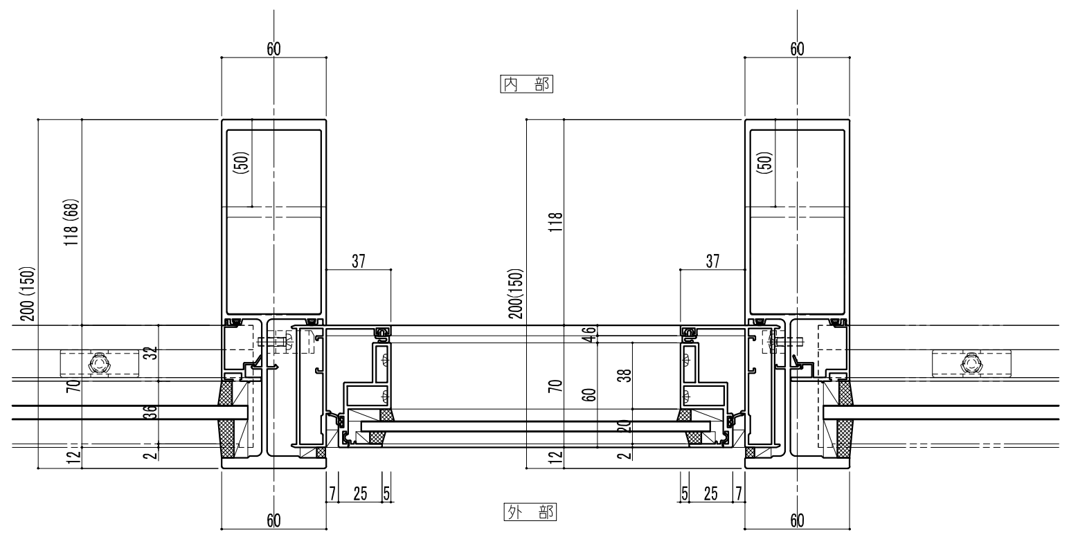
横断面図
