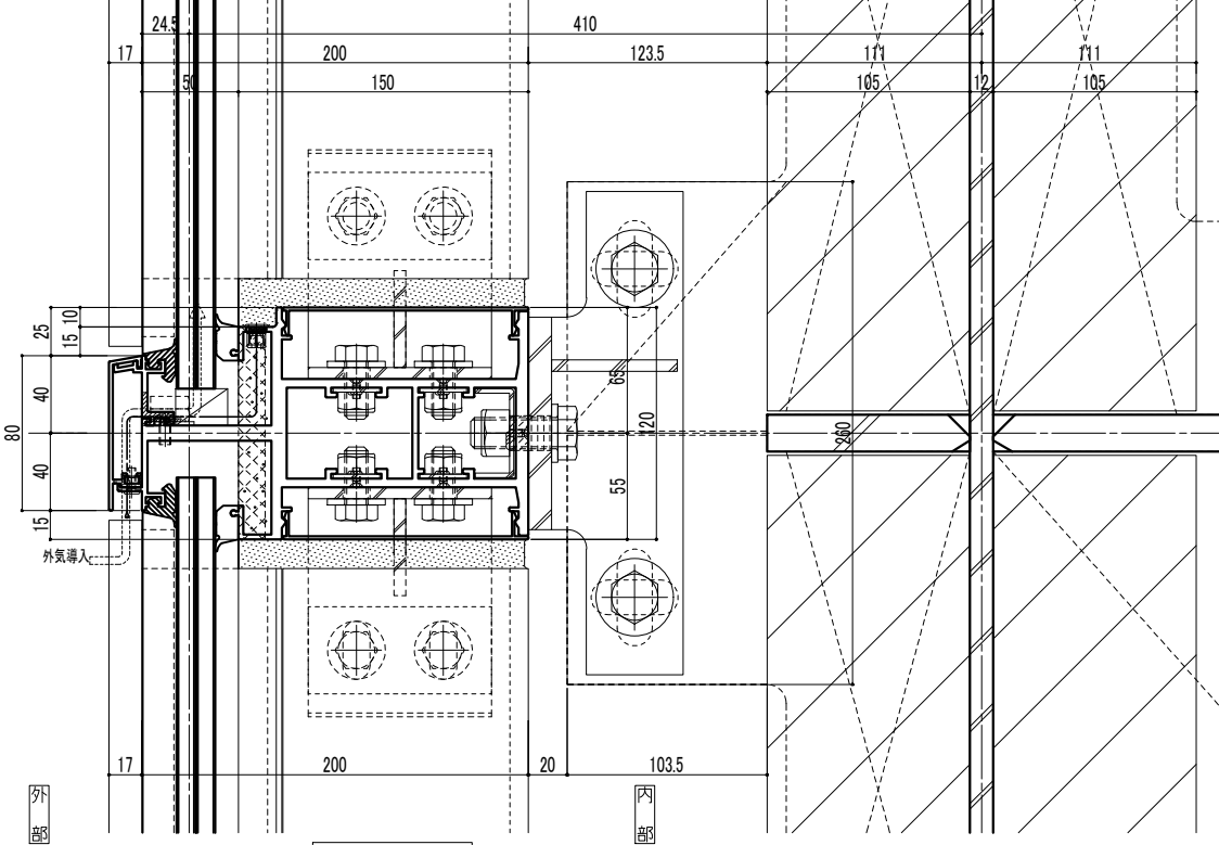
縦断図
