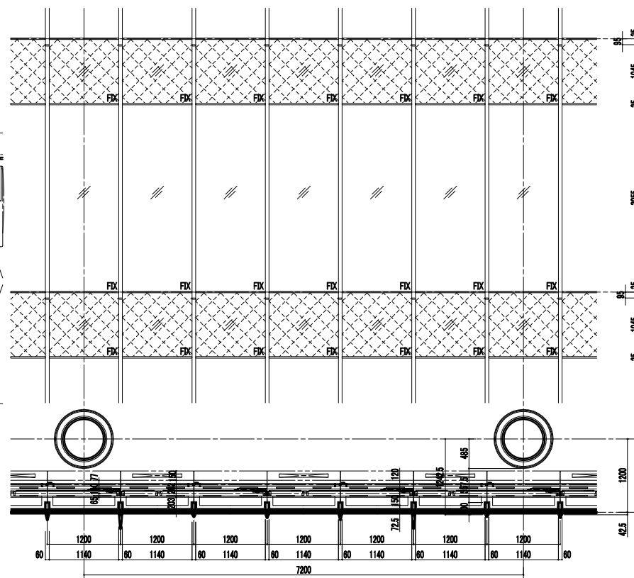
外観図
