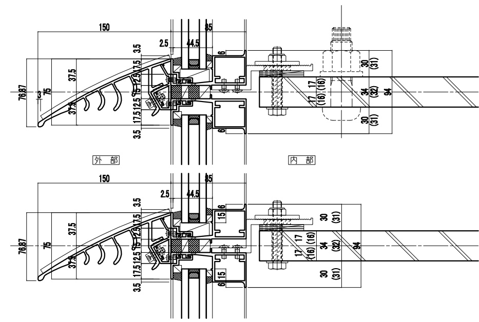
横断図
