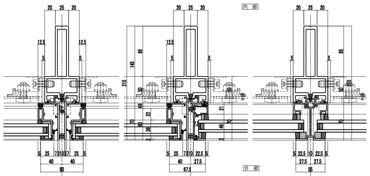
横断図
