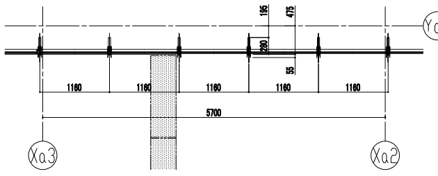
外観図
