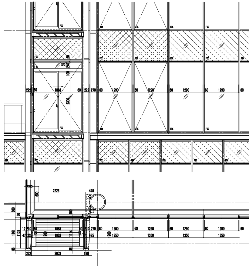
外観図
