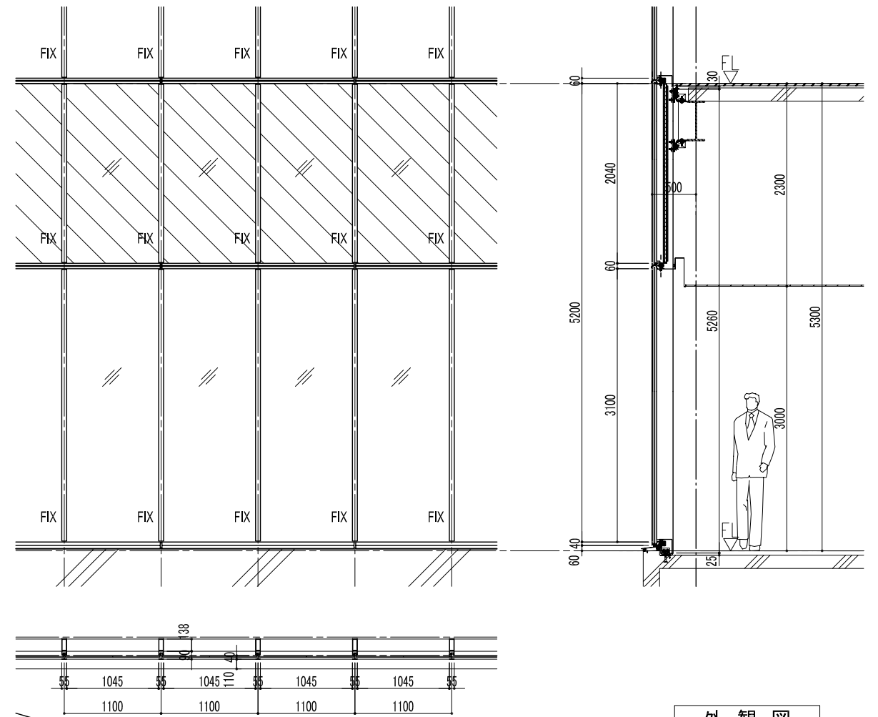
外観図
