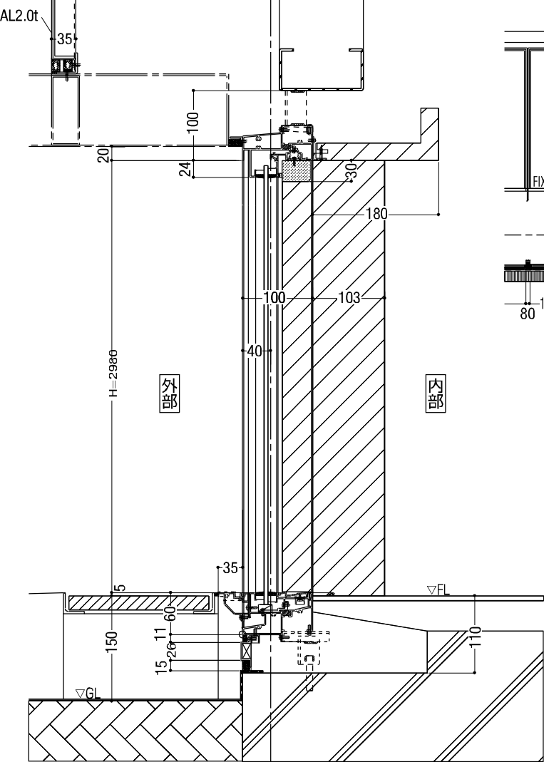
縦断面図
