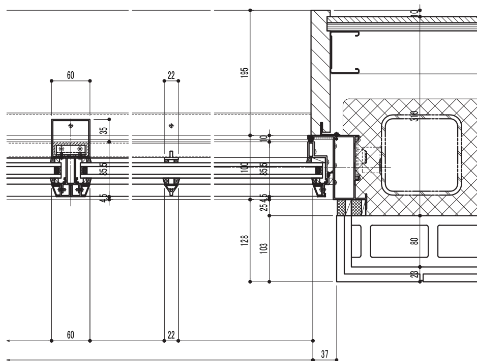
欄間排煙窓断面図
