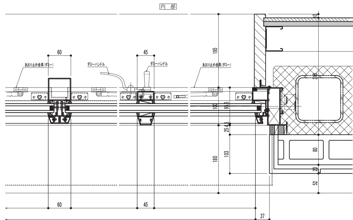
FIX窓断面図
