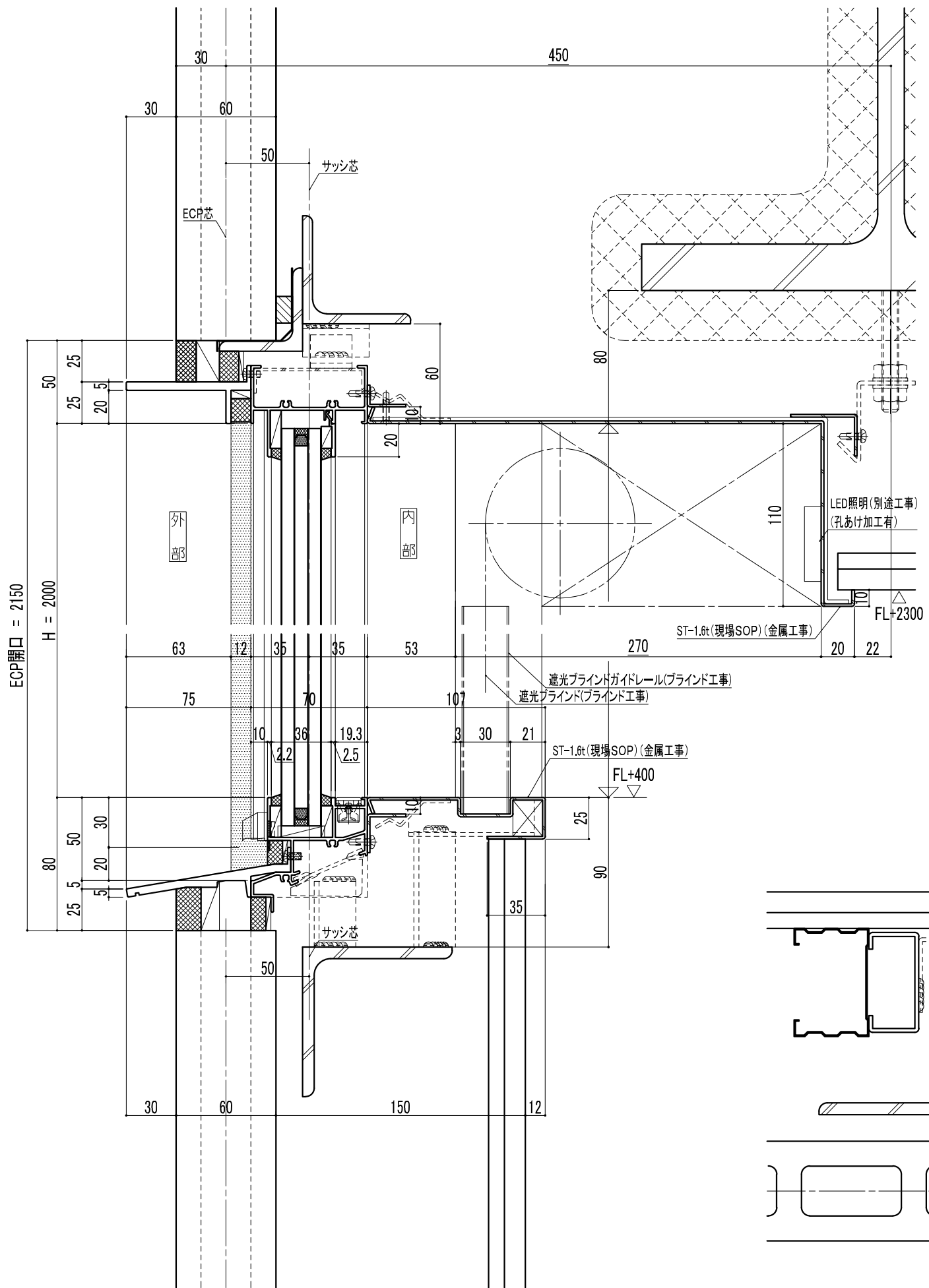
縦断図
