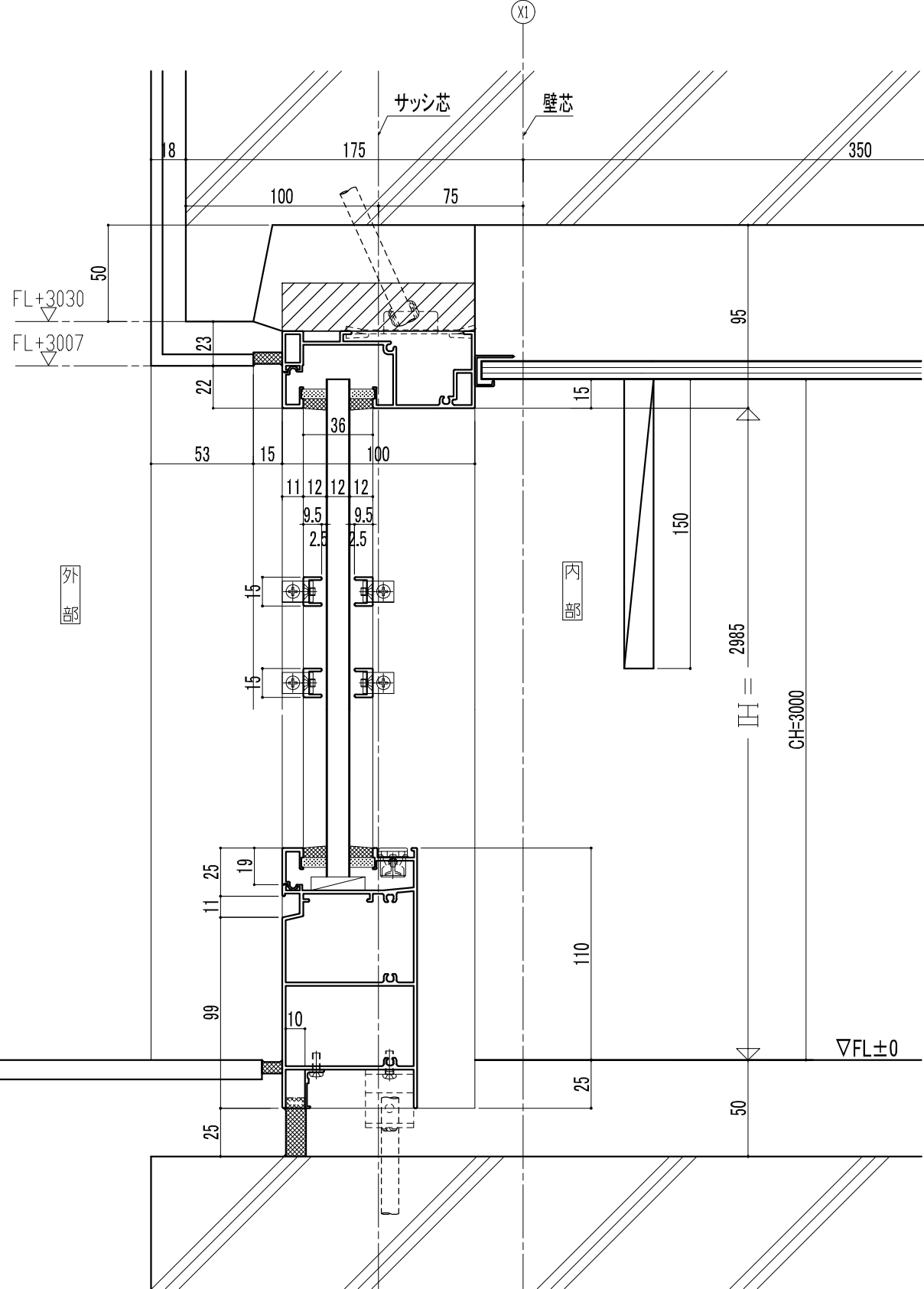
縦断図
