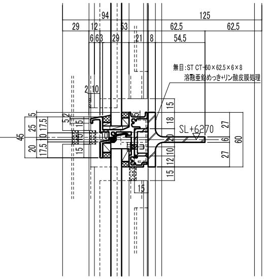
ホーム階防風スクリーン中間無目断面
