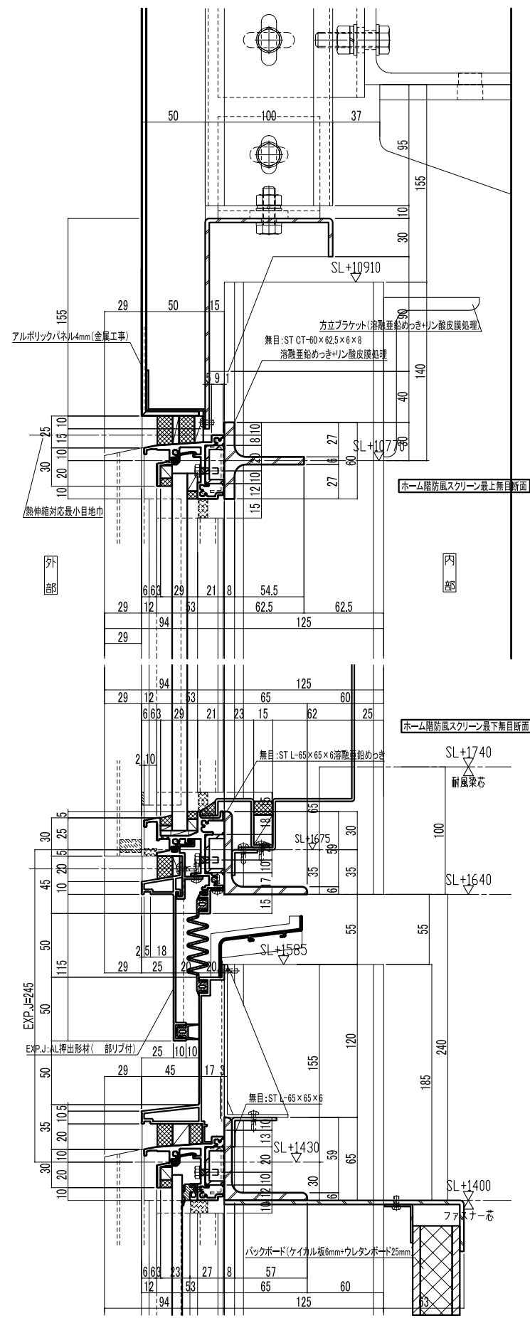
縦断図
