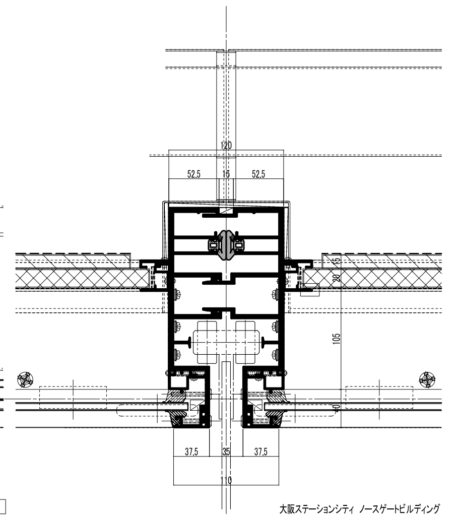
横断図
