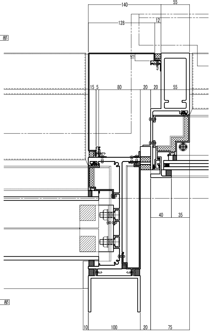
横断面図
