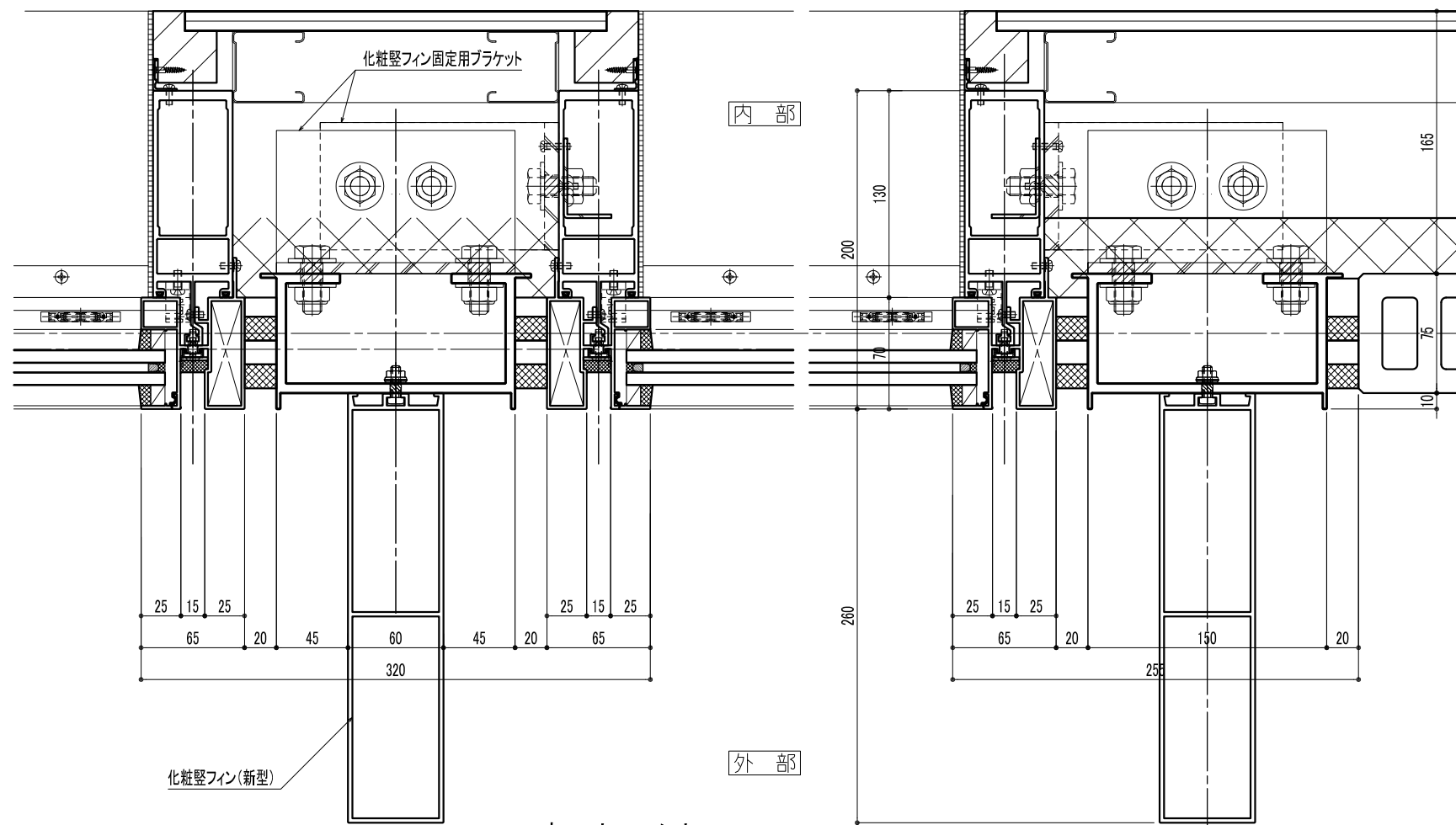
横断面図 (S=1/4)
