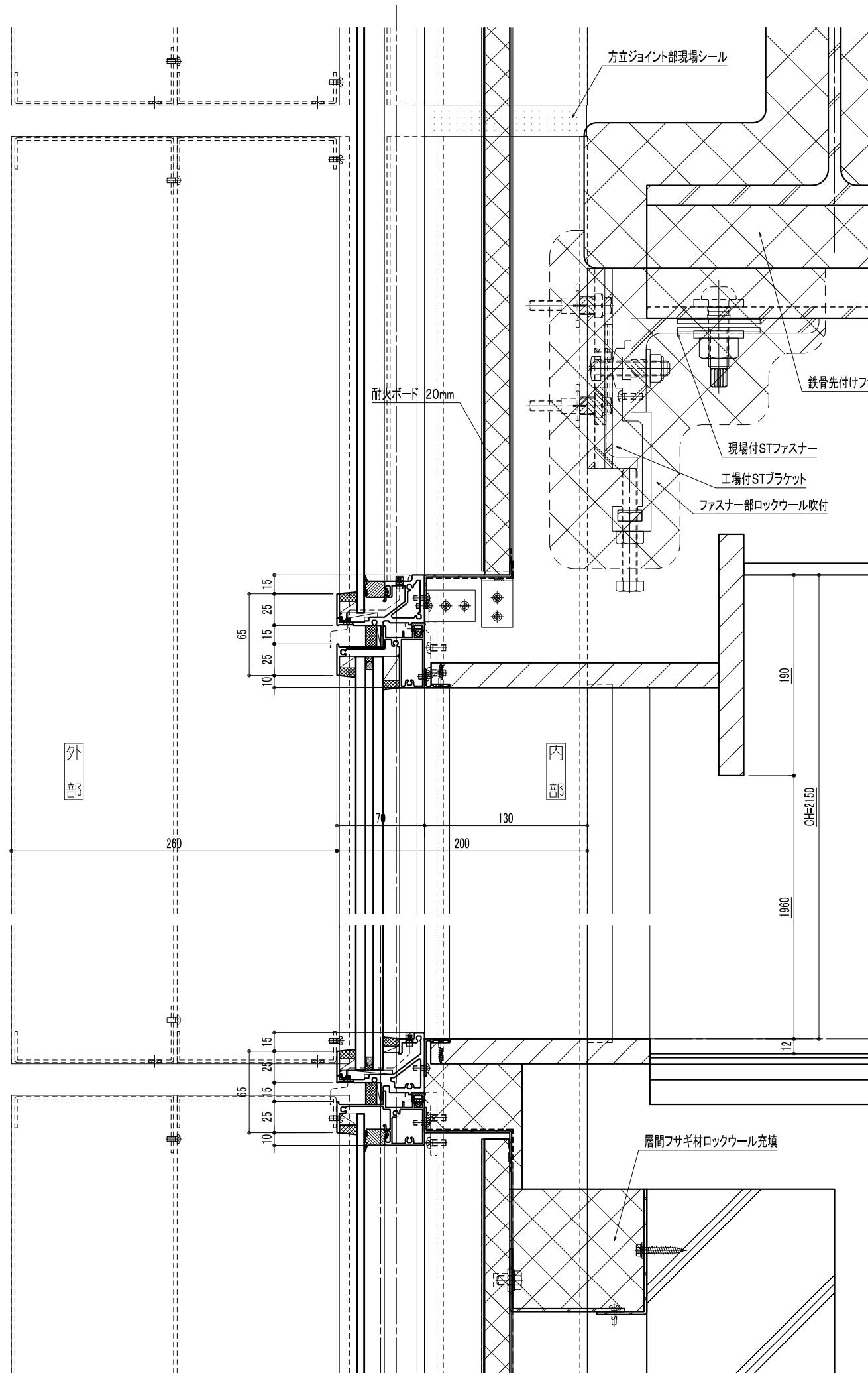
縦断面図 (S=1/4)
